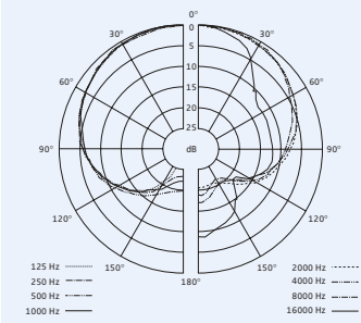
Polardiagramm MME 865-1
