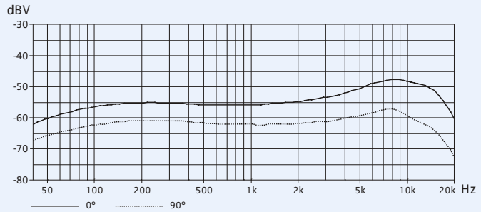
Frequenzgang MME 865-1
